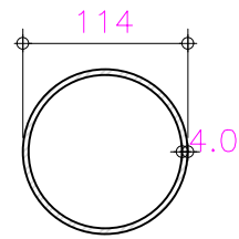
\text{Ø} = 4\frac{1}{2}'' \times 4.0\text{mm} PERFIL CIRCULAR ESCALA 1:10
