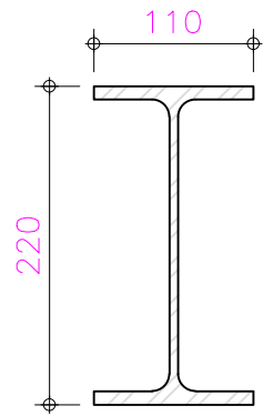
IPE 220 ESCALA 1:10
